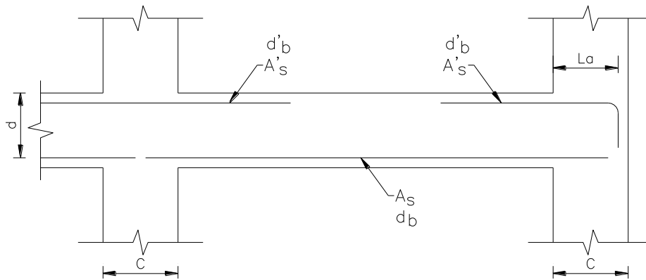
Figura 10.2 - Nomenclatura de áreas de acero y diámetros de barras
