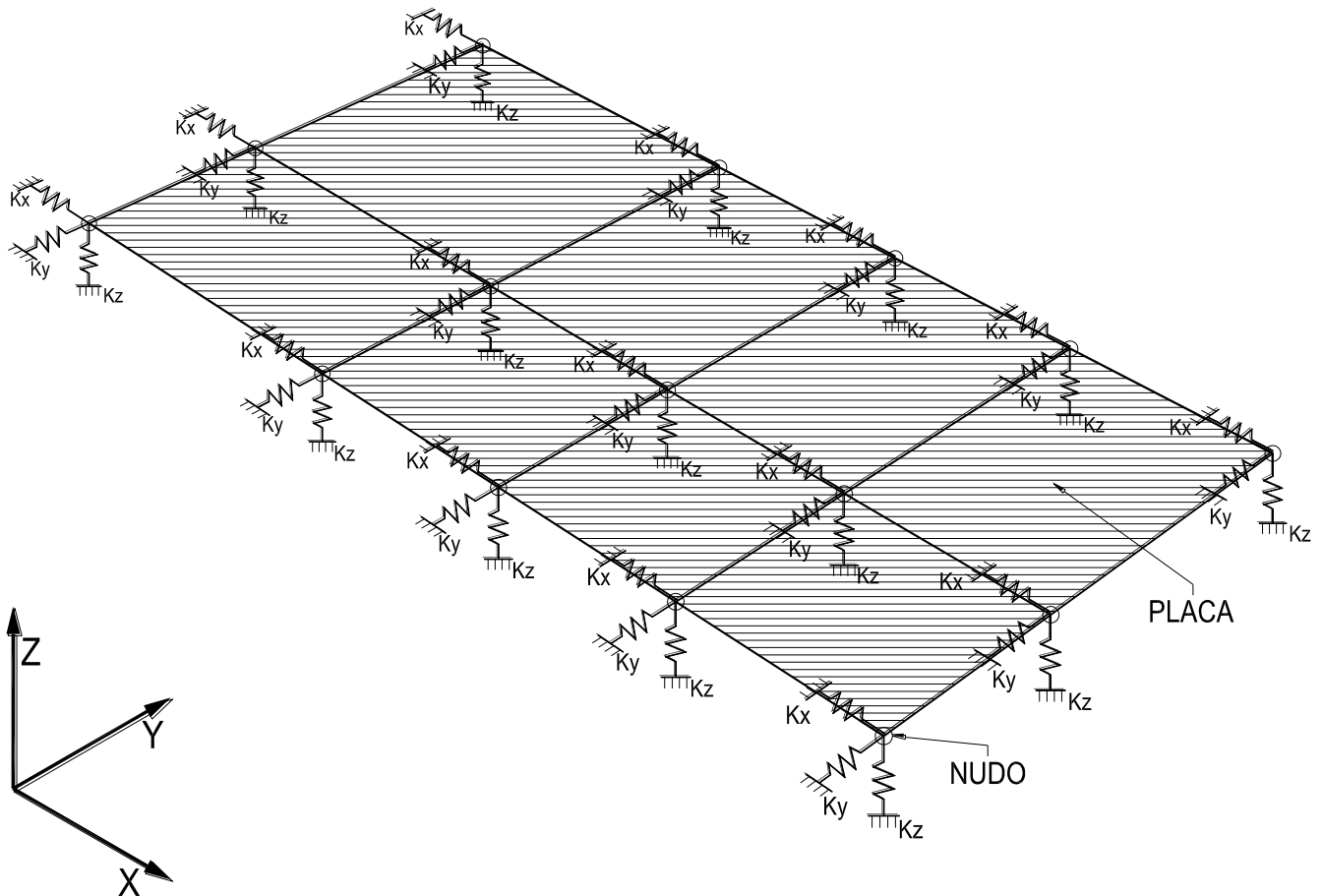
Figura 9.2 - Apoyos elásticos para losas
