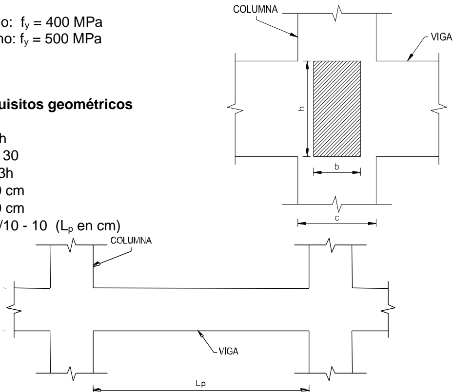
Figura 10.1 - Nomenclatura vigas y columnas
