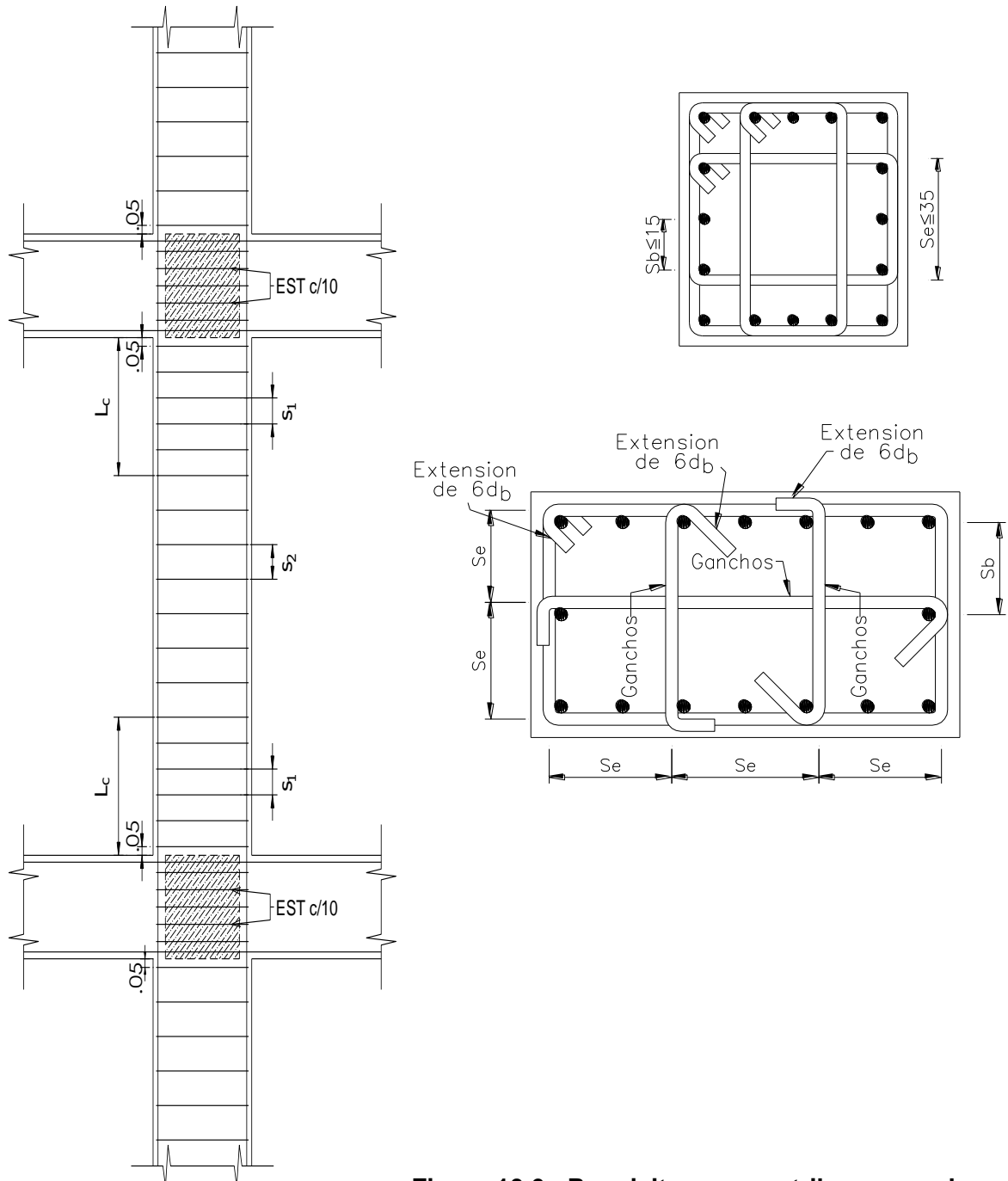
Figura 10.6 - Requisitos para estribos y ganchos
