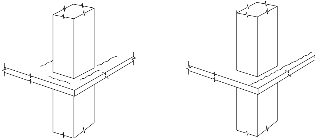
a) Grietas por Punzonamiento
