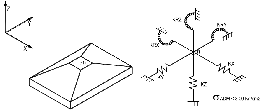
Figura 9.1 - Apoyos elásticos para zapatas
