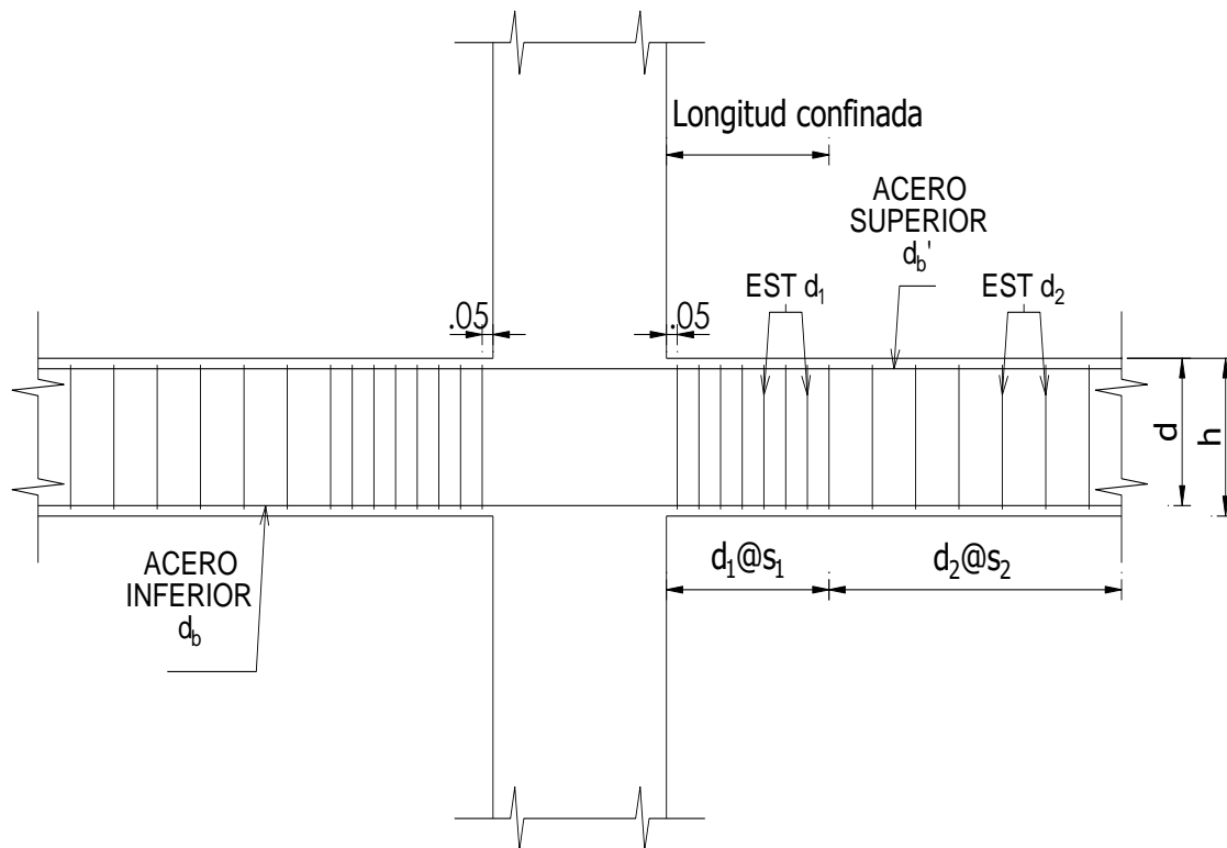
Figura 10.3 - Nomenclatura de refuerzos transversales
