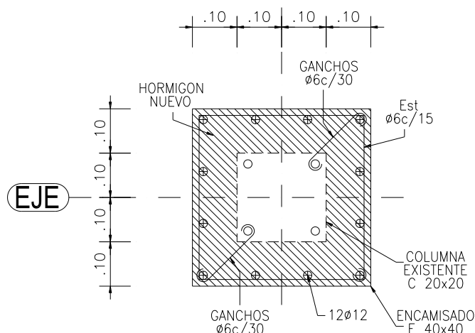
FIGURA FC11-6. ENCAMISADO DE COLUMNA
