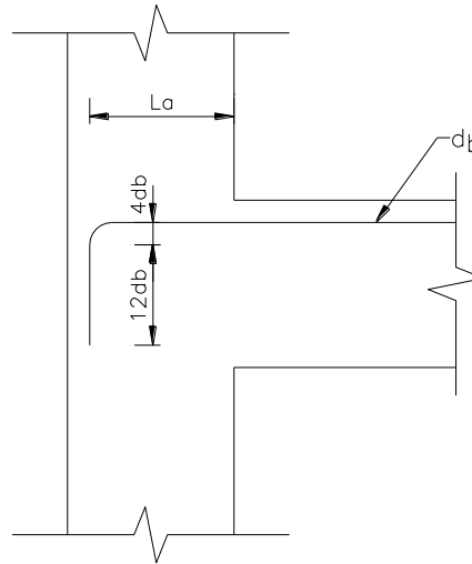
Figura 10.4 - Longitud de anclaje
