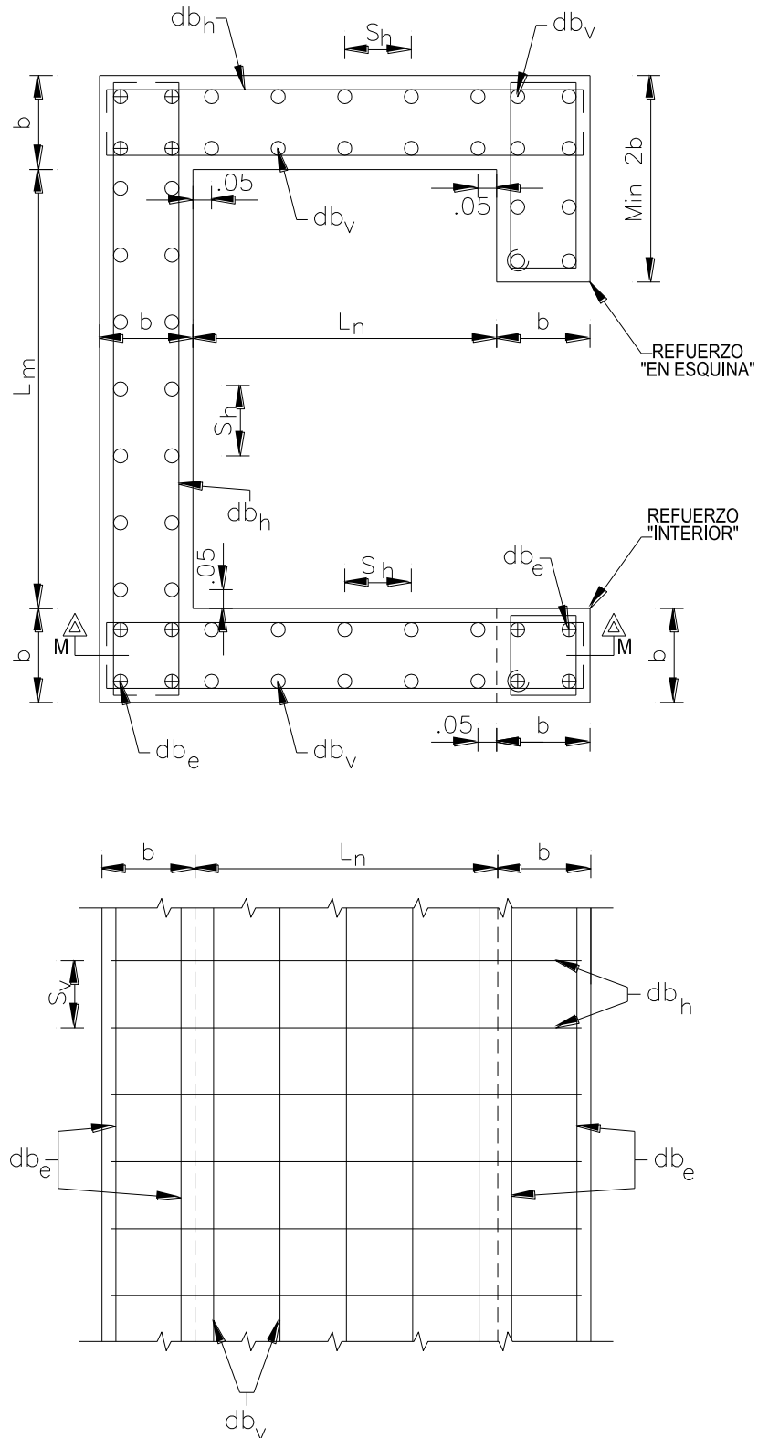
Figura 10.7 - Muros de cortante, vista en planta y sección M-M
