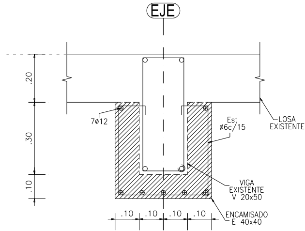
FIGURA FC11-7. ENCAMISADO DE VIGA
