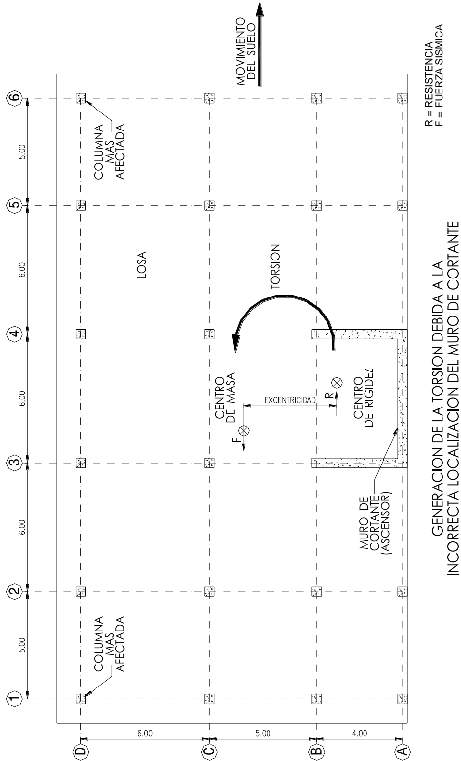
Figura 4.2 - Torsión generada por la incorrecta localización de muros de cortante
