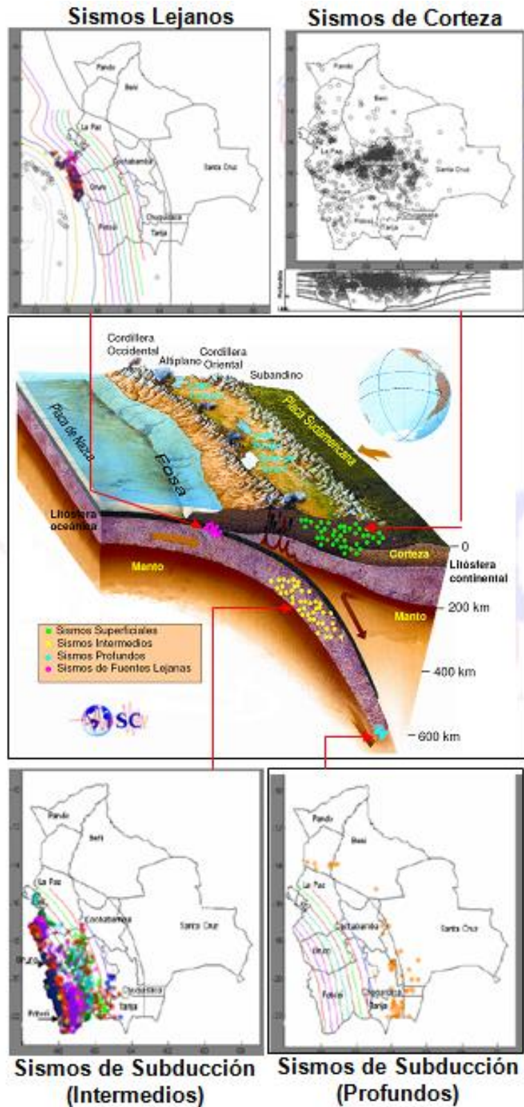
Figura 1 - Placas de Nazca y Sudamérica (Lamb S. and D. Sington, 1998 y Fuentes sismo génicas de Bolivia definidas de acuerdo a su origen)
