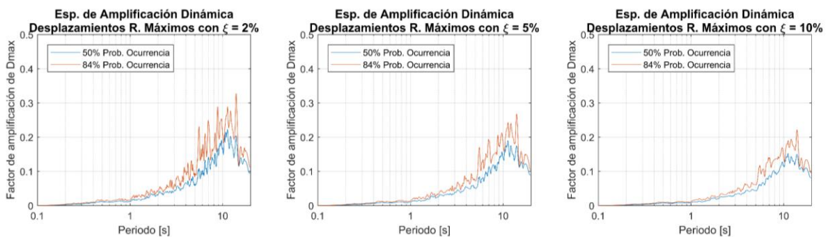
Figura 6-3. Espectros de amplificación dinámica de desplazamientos máximos.
