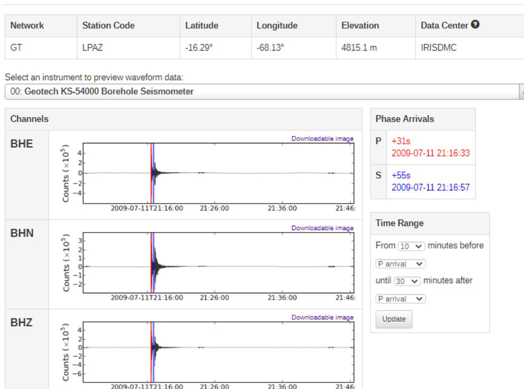
Figura A2.2. Ejemplo de registro sísmico en bruto.
