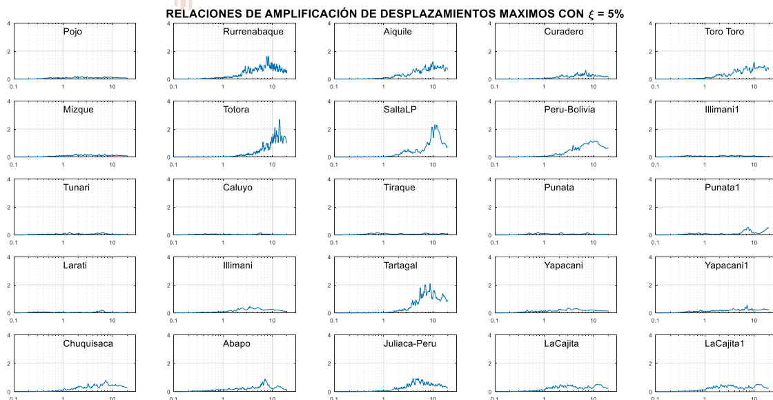
Figura A2.4. Envoltente de Espectros de respuesta desplazamientos normalizados.
