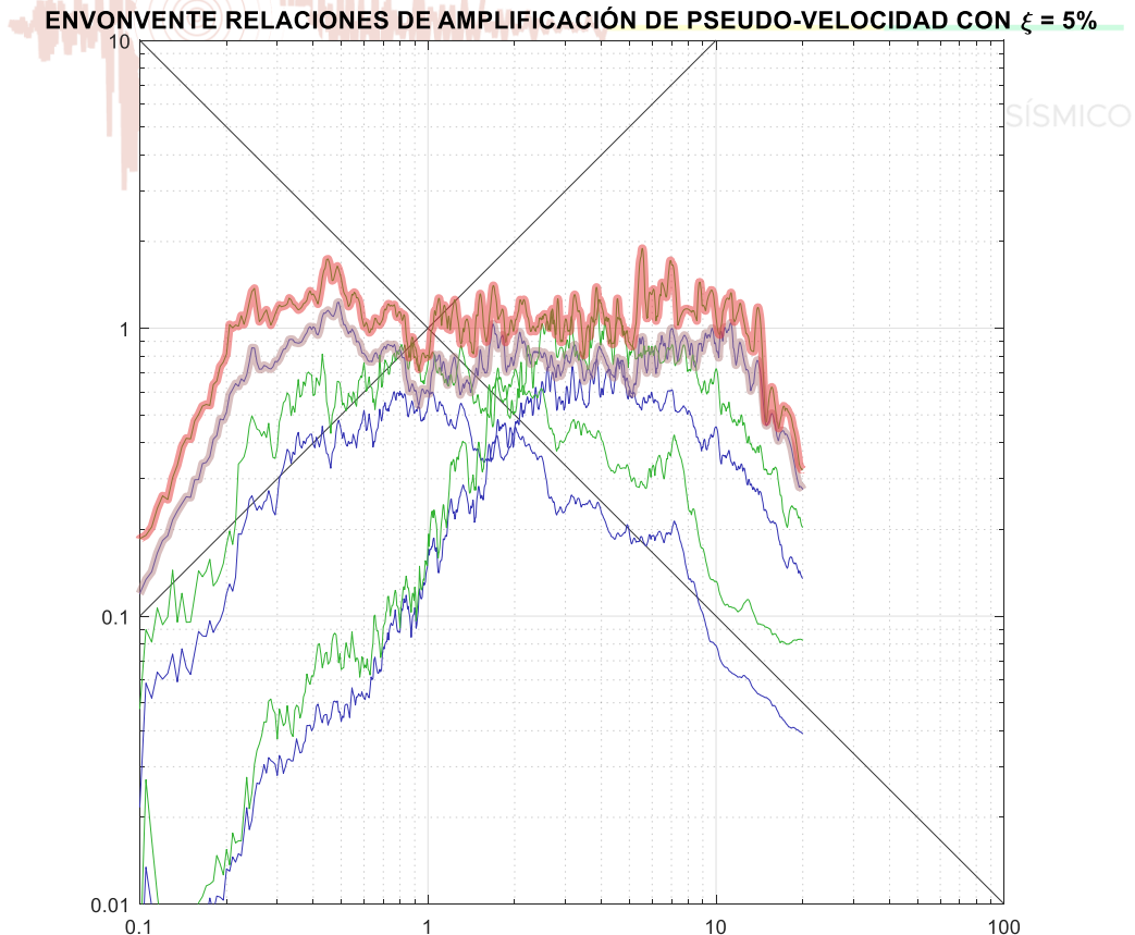
Figura A2.7. Envolvente total de los espectros de respuesta de pseudovelocity normalizados.
