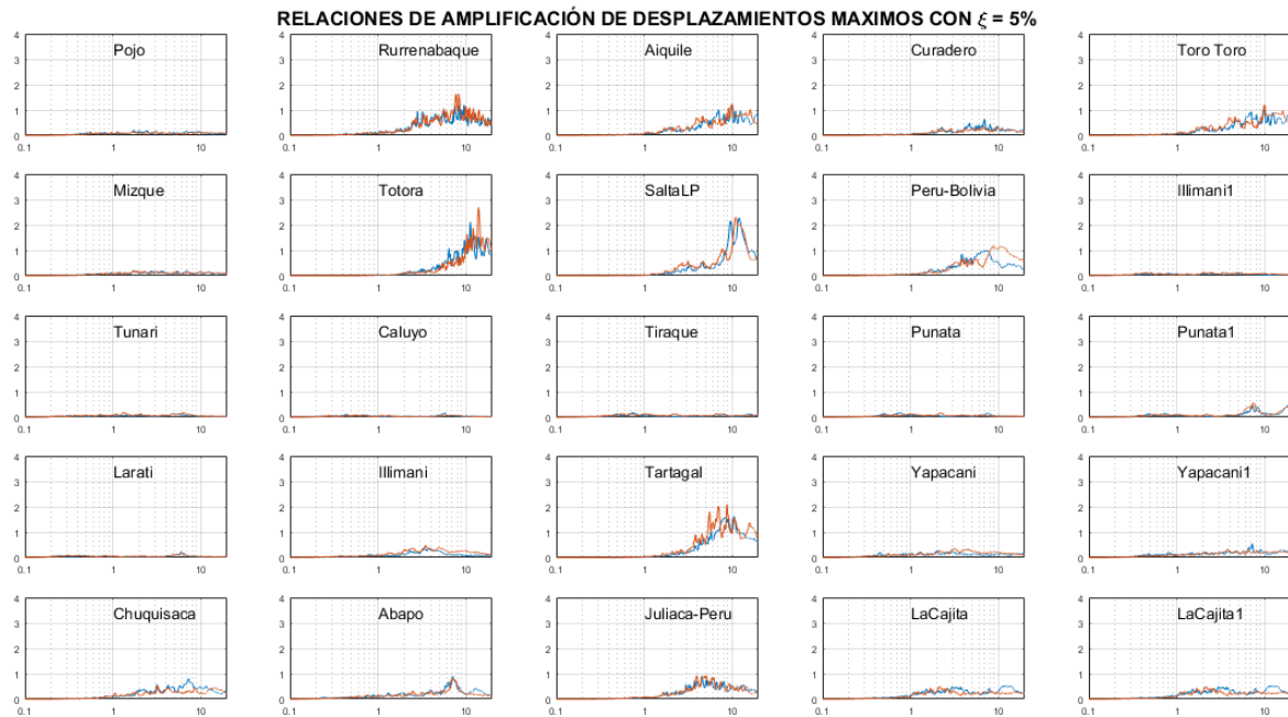
Figura A2.3. Espectros de respuesta de desplazamientos máximos normalizados aplicando la integral de Duhamel, sentido EO (azul) y NS (naranja).
